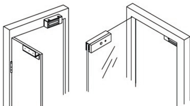
LZ支架安裝 (適用於門扇內開)
